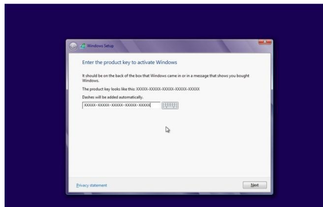
Perjanjian Lisensi
