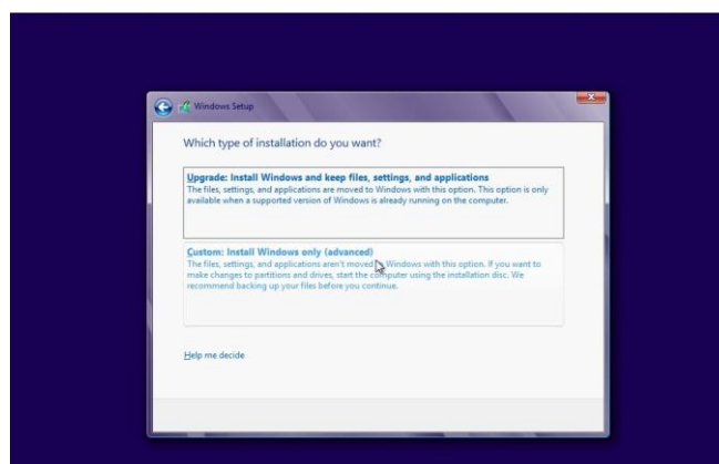
Tipe Instalasi
