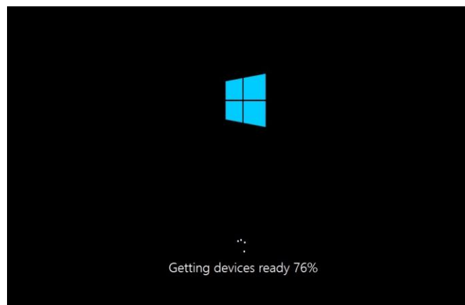
Intro Instalasi
