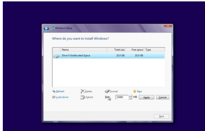
Pemartisi Harddisk
